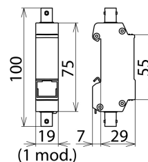
Rysunek wymiarowy DGA BNC VCD
