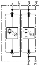
Schemat połączeń DV M TT 2P 255
