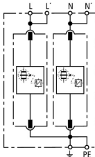
Schemat połączeń DV M TN 255
