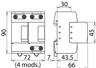
Rysunek wymiarowy DV M TN 255
