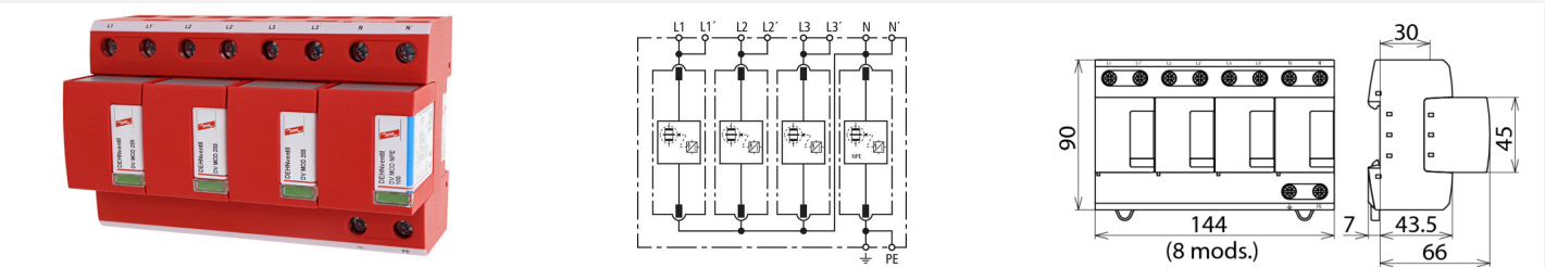
Ilustracje nie są wiążące Schemat połączeń DV M TT 255 Rysunek wymiarowy DV M TT 255 Kombinowany ogranicznik przepięć z modułami wymiennymi do sieci TT i TNS o napięciu znamionowym 230 / 400 V (układ połączeń "3+1").
