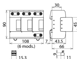
Rysunek wymiarowy DV M TNC 255 FM
