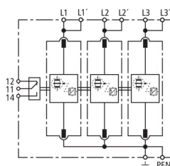
Schemat połączeń DV M TNC 255 FM
