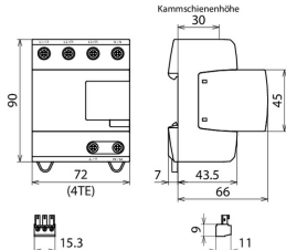
Rysunek wymiarowy DV M2 TNS 255 FM
