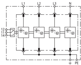
Schemat połączeń DV M2 TNS 255 FM
