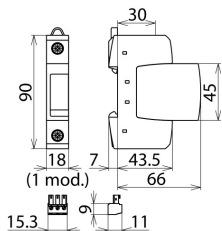
Rysunek wymiarowy DG S 385 VA FM
