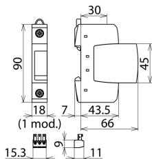
Rysunek wymiarowy DG S 75 VA FM
