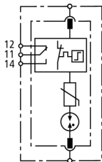
Schemat połączeń DG S 75 VA FM
