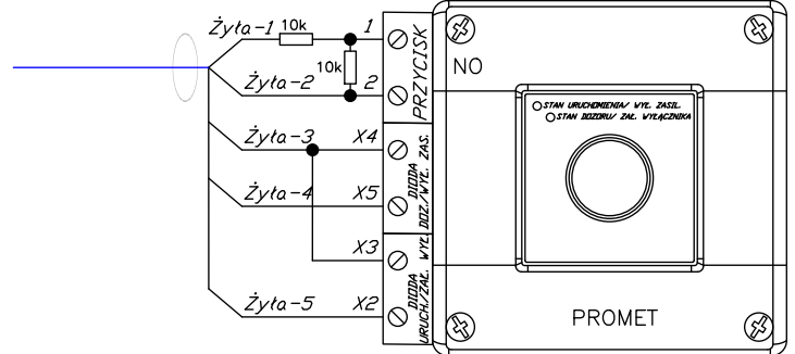
PWP URZĄDZENIE URUCHAMIAJĄCE
