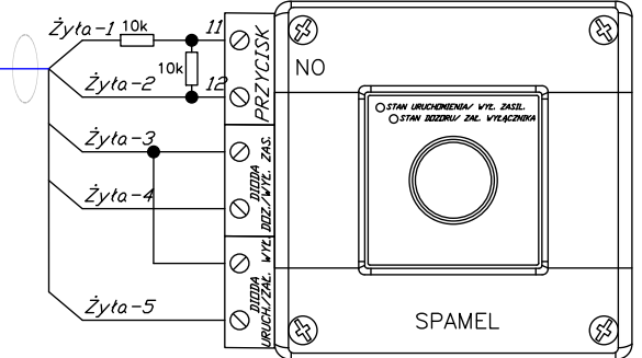
DETAL A PWP URZĄDZENIE URUCHAMIAJĄCE
