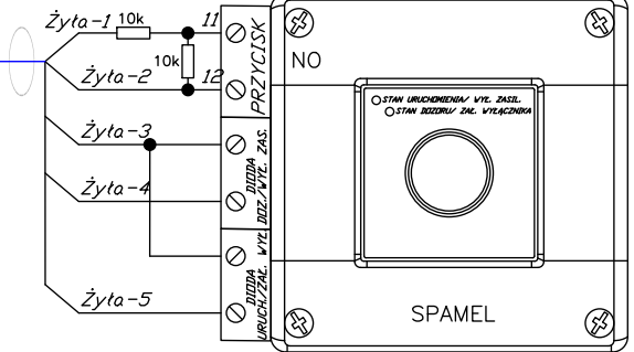
DETAL A PWP URZĄDZENIE URUCHAMIAJĄCE
