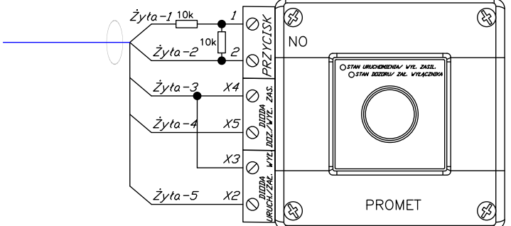
DETAL B PWP URZĄDZENIE URUCHAMIAJĄCE
