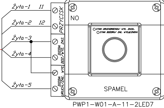
DETAL A PWP URZĄDZENIE URUCHAMIAJĄCE
