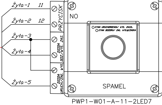
DETAL A PWP URZĄDZENIE URUCHAMIAJĄCE
