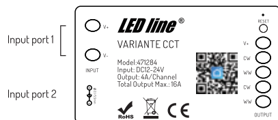
Abb.1 Controller-Ansicht
