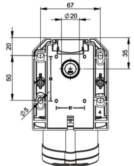
b=Höhe/height Neigung/angle=15°
