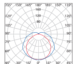
MIRA 2 × 36W
