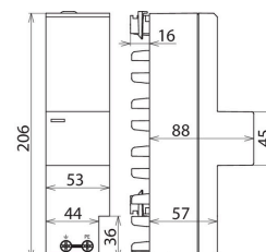
Dimensions DSH ZP B TT 255
