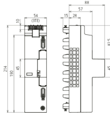
Dimension drawing DSH ZP 2 LSG TT 255
