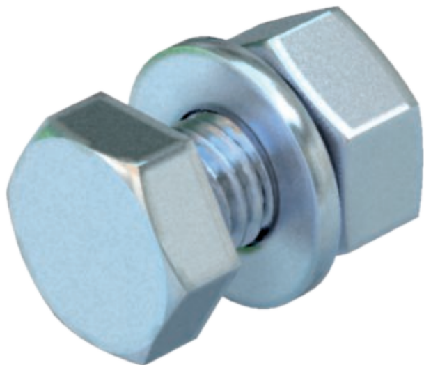
Śruba z łbem sześciokątnym z nakrętką i podkładką M8x30.
