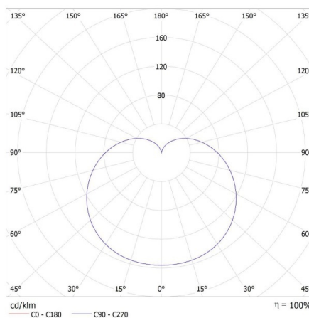
KANLUX S.A. (kat 33743) IQ-LED G45E27 7,2W-WW / LDC (Polar)
