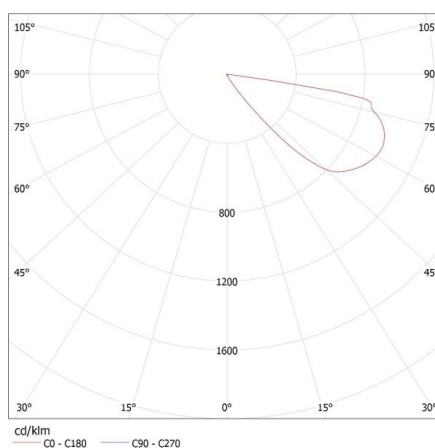
KANLUX S.A. (kat 22760) ONSTAR LED-GR / Krzywa rozsyłu światła (biegunowo)
